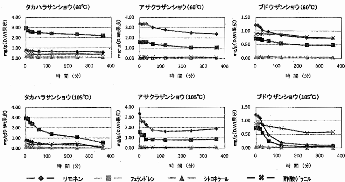
図-10 加熱 (60, 105°C) におけるテルペン含量変化
