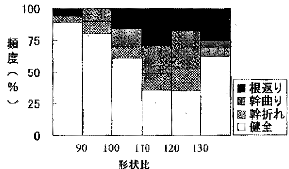
図-10 形状比階別被害形態頻度分布
