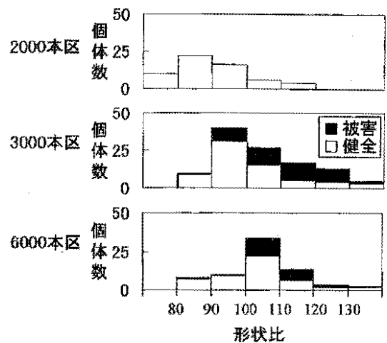
図-9 各試験区の形状比階分布
