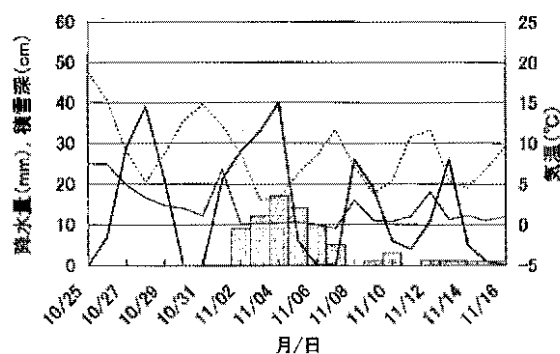
付図-5 長滝地域気象観測所における2002年10月下旬から11月上旬の気象 点線は最高気温、細実線は最低気温、太実線は降水量、棒は積雪深を示す。
