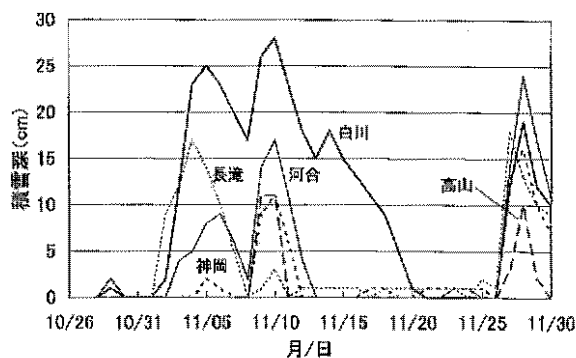
図-17 2002年10月下旬から11月における積雪深の推移
