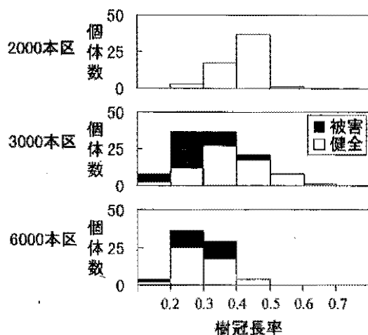
図-11 各試験区の樹冠長率階分布
